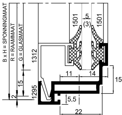
AANSLUITDETAIL ③
